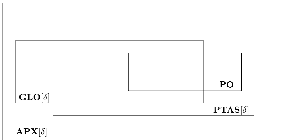
FIG. 1 – Les classes \mathbf{GLO}[\delta] et les classes d'approximation.
