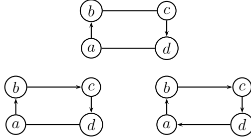
FIG. 11 – Configurations interdites dans une structure d'ordre d'intervalle
