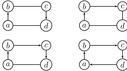
FIG. 9 – Configurations interdites dans une structure de semi-ordre
