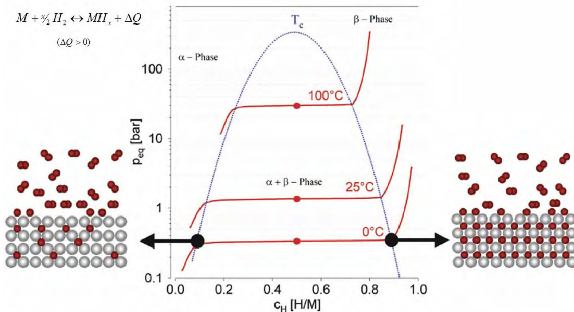
Figure 7 : Représentation schématique et diagramme PCT caractéristique du mécanisme d'hydruration [7].
