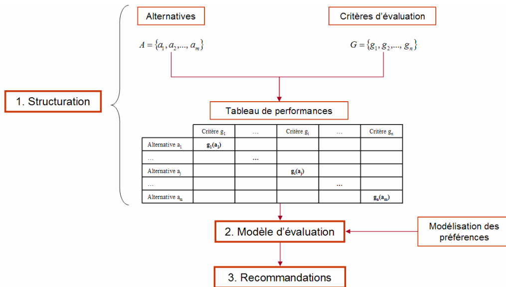
Figure 11 : Vue d'ensemble des étapes qui interviennent dans un processus d'aide à la décision multicritère.
