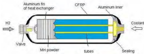
Figure 8 : Réservoir de stockage solide développé par le constructeur automobile TOYOTA. L'hydrure employé est de type TiCrMn [8].
