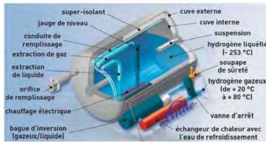
Figure 5 : Représentation schématique d'un réservoir d'hydrogène liquide du fabricant Linde [3].
