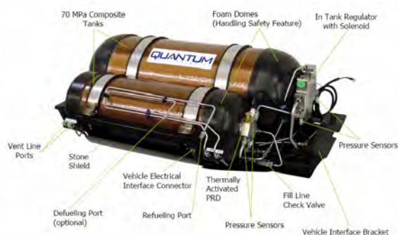
Figure 3 : Système de stockage d'hydrogène à 70 MPa développé par la société Quantum. La capacité de stockage de ce système est de 3,1 kg [5].
