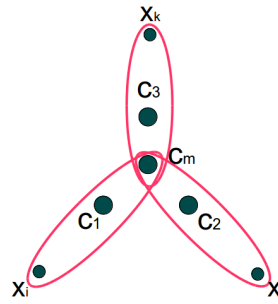
Fig. 6. The clause gadget
