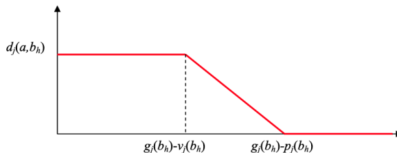
Figure 4. Détermination de l'indice de discordance
