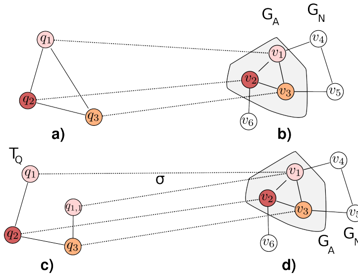
FIGURE 3.3 – Illustration de l'alignement effectué par PADA1. Le graphe requête de départ est en a), il est transformé en arbre avec un sommet dupliqué, en c). Le réseau G_N dans lequel est effectuée la requête est présenté en b) et d). La fonction \sigma donne les sommets du réseau étant alignés avec les sommets de la requête. Comme q_1 et q_{1,1} représentent le même sommet q_1 dans le graphe de départ, ils doivent être alignés avec le même sommet dans le réseau. Le sous-graphe du réseau correspondant à la requête est nommé G_A .
